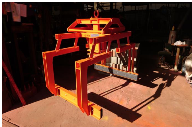
G70-B8-12 (空洞ブロック 3 段用)
